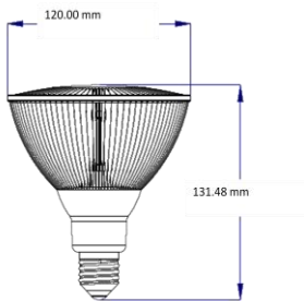
E26/27(EURO) Beam Angle 38°,72° ,120°,135°
