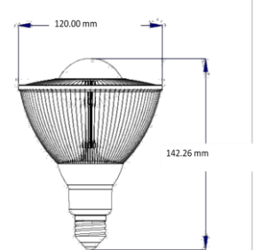
E26/24(US) Beam Angle 100°
